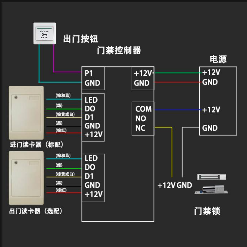
接控制板接线图
