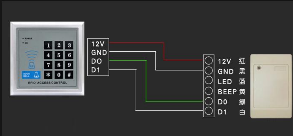
接一体机、考勤机接线图
